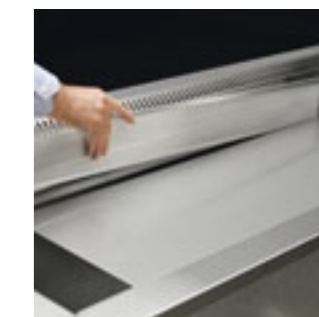
Facile pulizia ed igiene del vano evaporatore Evaporator compartment easy to inspect and to clean
